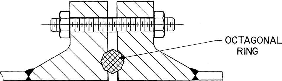
Fig. 3.3.4. Ring joint.
